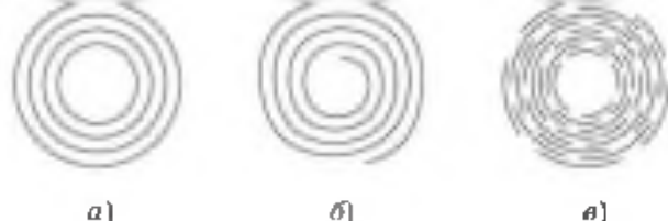
Рис. 149. Варианты поперечного разреза нанотрубок: а — «ругбейская матрица»; б — «рулонный свёрток»; в — «папье-маше»
