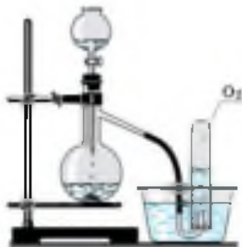
Рис. 60. Получение кислорода в лаборатории разложением пероксида водорода и собирание его методом вытеснения воды
