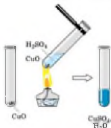
Рис. 130. Взаимодействие оксида меди (II) с сервой кислотой
