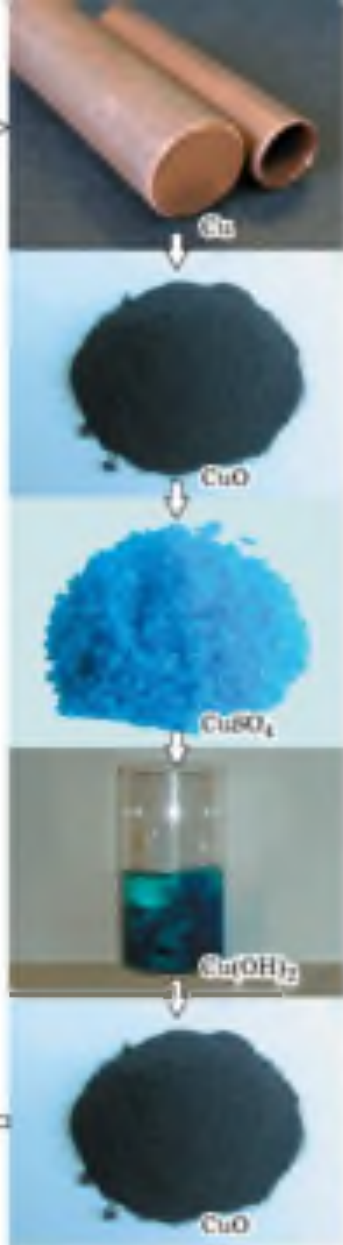
Рис. 147. Генетический ряд меди
