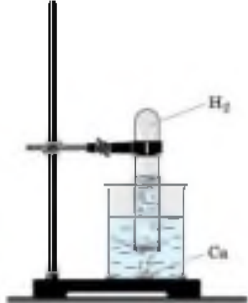
Рис. 118. Взаимодействие кальция с водой
