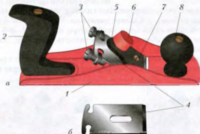
Рис. 34. Рубанок с металлической колодкой: а — общий вид; 1 — колодка; 2 — рукоятка; 3 — регулировочные винты; 4 — нож; 5 — стружколоматель; 6 — зажимной винт; 7 — винт; 8 — ручка; 9 — лезвие
