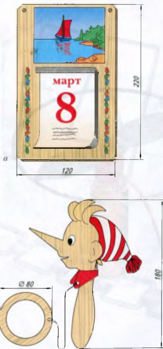
Рис. 174. Подвеска для отрывного календаря (материал – фанера) (а); игра «Набрось кольцо на нос» (б)
