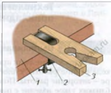
Рис. 70. Выпиловочный столик: 1 – верстак; 2 – струбцина; 3 – дощечка
