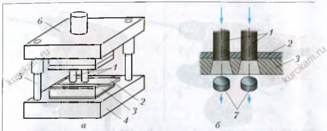
Рис. 138. Общий вид штампа (а) и процесс пробивания отверстий (б):
