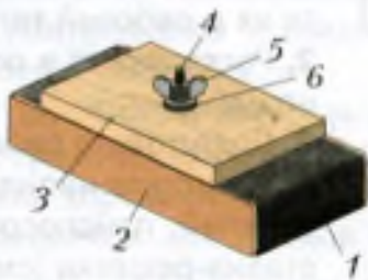
Рис. 64. Шлифовальная колодка: 1 – шлифовальная шкурка; 2 – корпус; 3 – прижимная планка; 4 – винт; 5 – зажимная гайка; 6 – шайба
