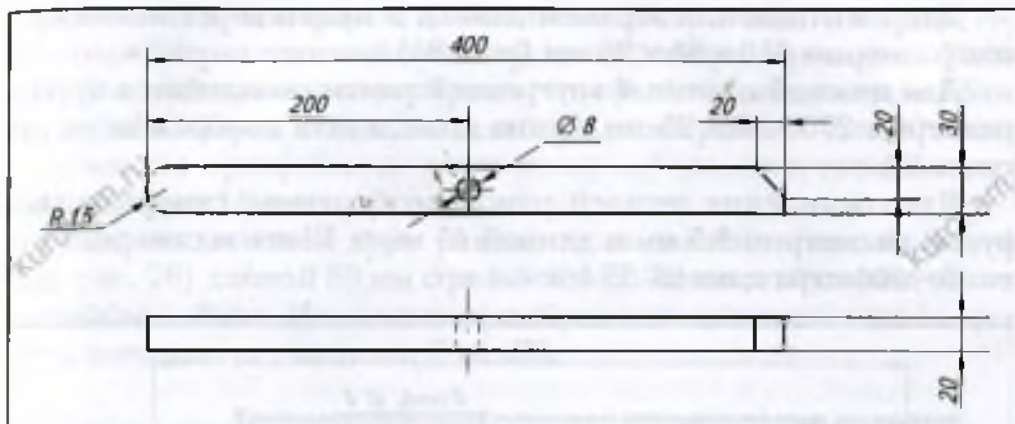
Рис. 79. Эскиз ножки 1
