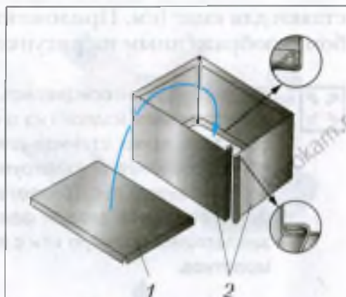
Рис. 153. Общий вид металлической коробки с соединением боковых стенок фальцевым швом: 1 – дно; 2 – боковые стенки
