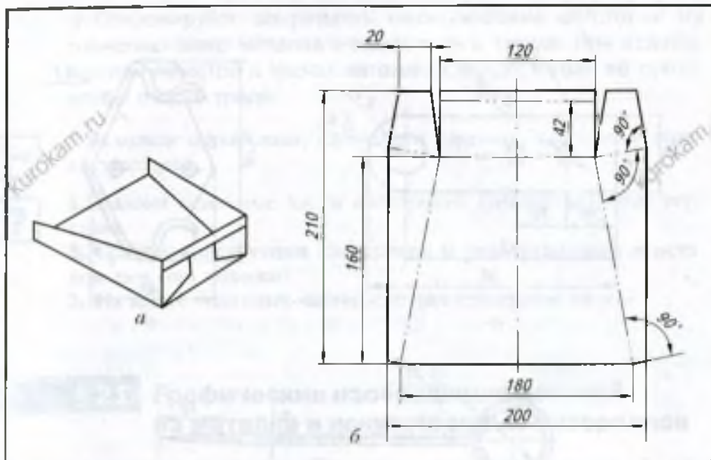
Рис. 98. Корпус хозяйственного совка: а – технический рисунок; б – чертёж развёртки
