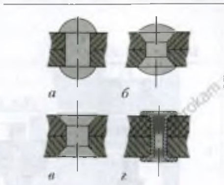
Рис. 145. Виды заклёпок: а – с полукруглой головкой; б – с полупотайной головкой; в – с потайной головкой; г – трубчатая
