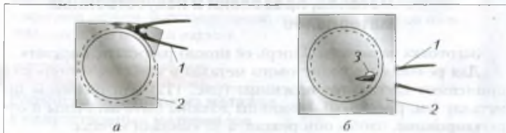
Рис. 114. Вырезание круга (а) и отверстия (б): 1 – слесарные ножницы; 2 – заготовка; 3 – технологическое отверстие
