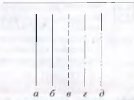
Рис. 13. Линии чертежа: а — сплошная основная; б — размерная или выносная; в — штриховая; г — штрихпунктирная; д — штрихпунктирная с двумя точками
