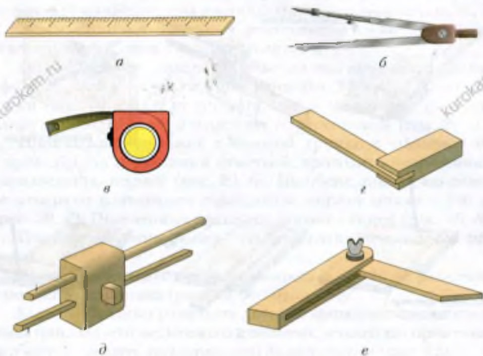
Рис. 19. Инструменты для разметки заготовок из древесины: а – линейка; б – циркуль; в – рулетка; з – столярный угольник; д – рейсмус; е – малка
