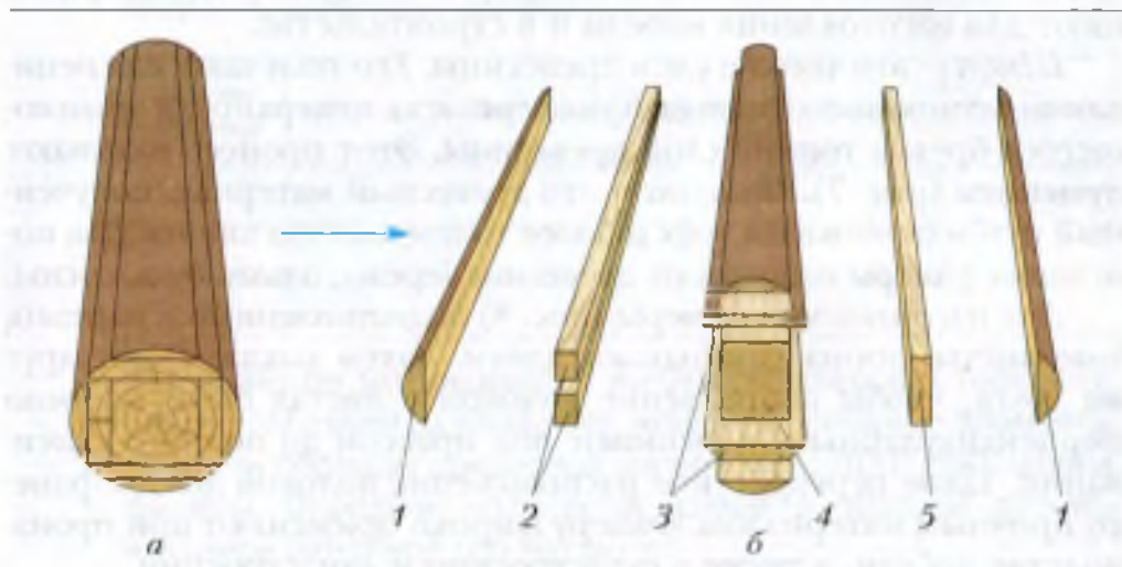
Рис. 5. Виды пиломатериалов: a – бревно с разметкой; б – виды пиломатериалов: 1 – горбыль; 2 – бруски; 3 – доска необрезная; 4 – брус; 5 – доска обрезная
