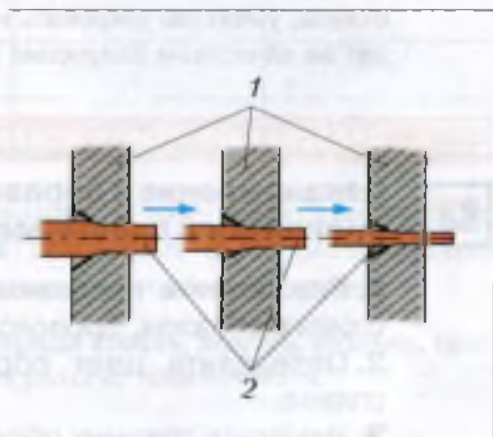
Рис. 91. Схема получения проволоки волочением: 1 – фильеры; 2 – проволока
