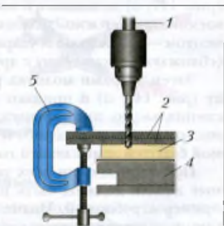
Рис. 146. Сверление отверстий под заклёпку: 1 – шпиндель сверлильного станка; 2 – детали; 3 – деревянный брусок; 4 – стол станка; 5 – струбцина
