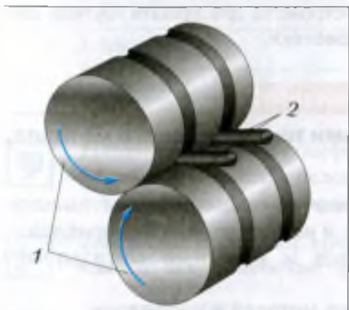
Рис. 90. Схема прокатки проволоки: 1 – валки; 2 – проволока
