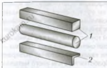
Рис. 125. Металлические элементы для гибки заготовок в тисках: 1 – оправки; 2 – уголок
