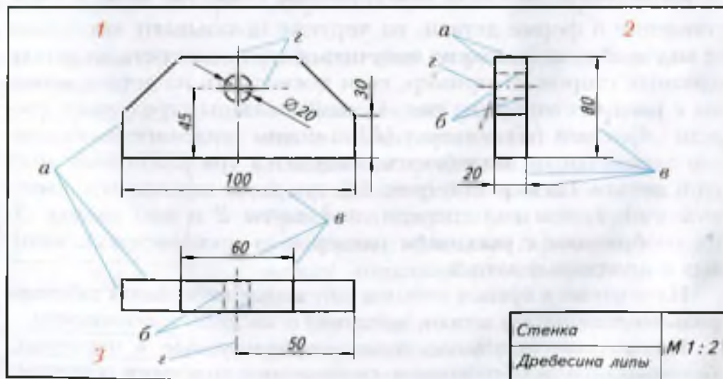
Рис. 12. Чертёж детали «стенка»: 1 – главный вид; 2 – вид слева; 3 – вид сверху: а – основные линии; б – птриховые линии; в – размерные и выносные линии; г – птрихпунктирные линии
