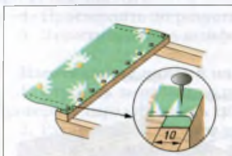
Рис. 87. Крепление сиденья
