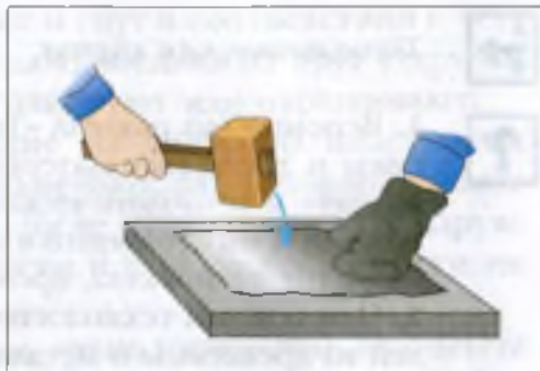
Рис. 105. Правка тонколистовой заготовки киянкой
