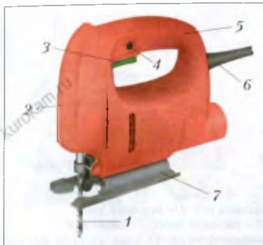
Рис. 30. Электрелобзик: 1 – пила; 2 – корпус; 3 – кнопка включения; 4 – кнопка блокировки включения; 5 – ручка; 6 – электрический шнур; 7 – опора
