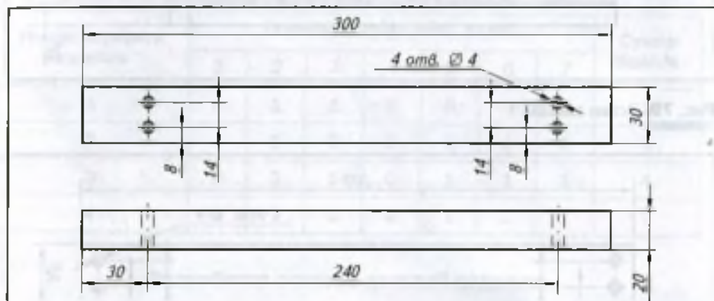
Рис. 81. Эскиз верхней планки 3
