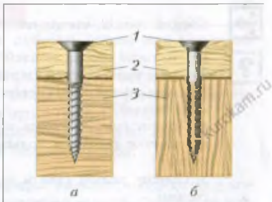
Рис. 55. Соединение деталей шурупами поперёк волокон (а) и вдоль волокон (б) основной детали: 1 – шуруп; 2 – присоединяемая деталь; 3 – основная деталь
