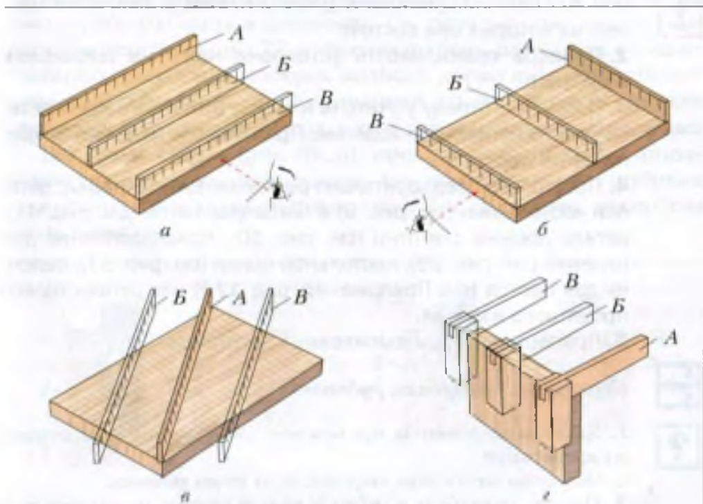
Рис. 37. Проверка прямолинейности отстроганной пласти заготовки (а — в) и перпендикулярности кромки относительно пласти (г)
